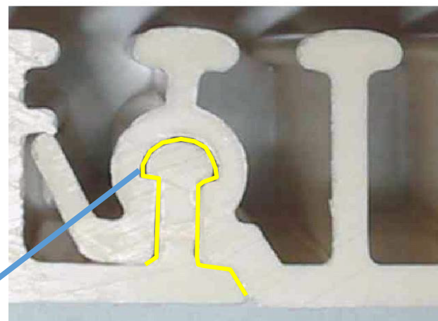
かん合状況
